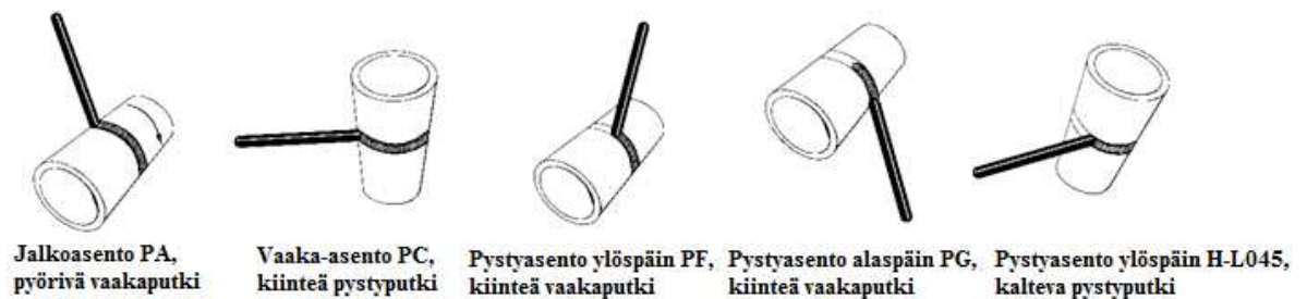
Kuva 5. Päittäishitsiasennot putken hitsauksessa [3].
