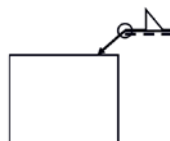
Kun kappale on ympärihitsattava, käytetään ympyrätunnusta
